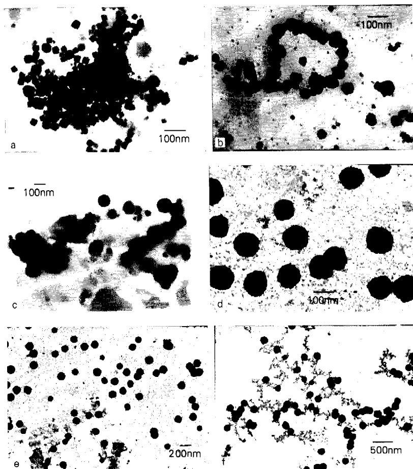
图5 富集液中高密度颗粒的电镜观察
