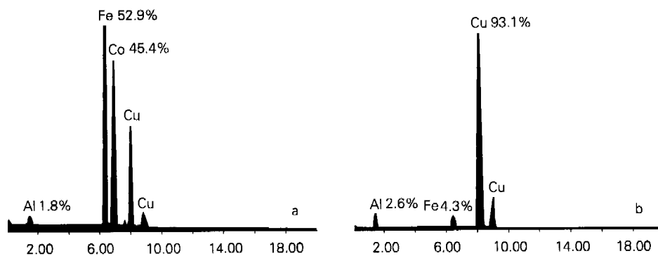
图6 富集液中致密颗粒的能谱分析
