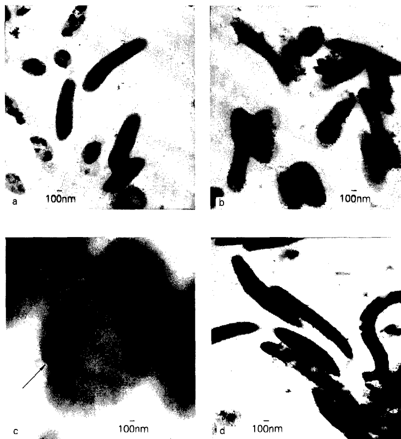
图 4 富集液中细菌的电镜观察
