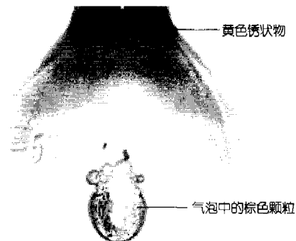
图2 趋磁细菌的富集
